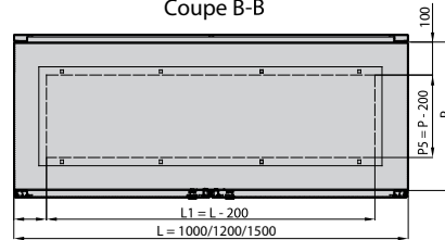
Coupe B-B
