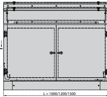
Coupe B-B
